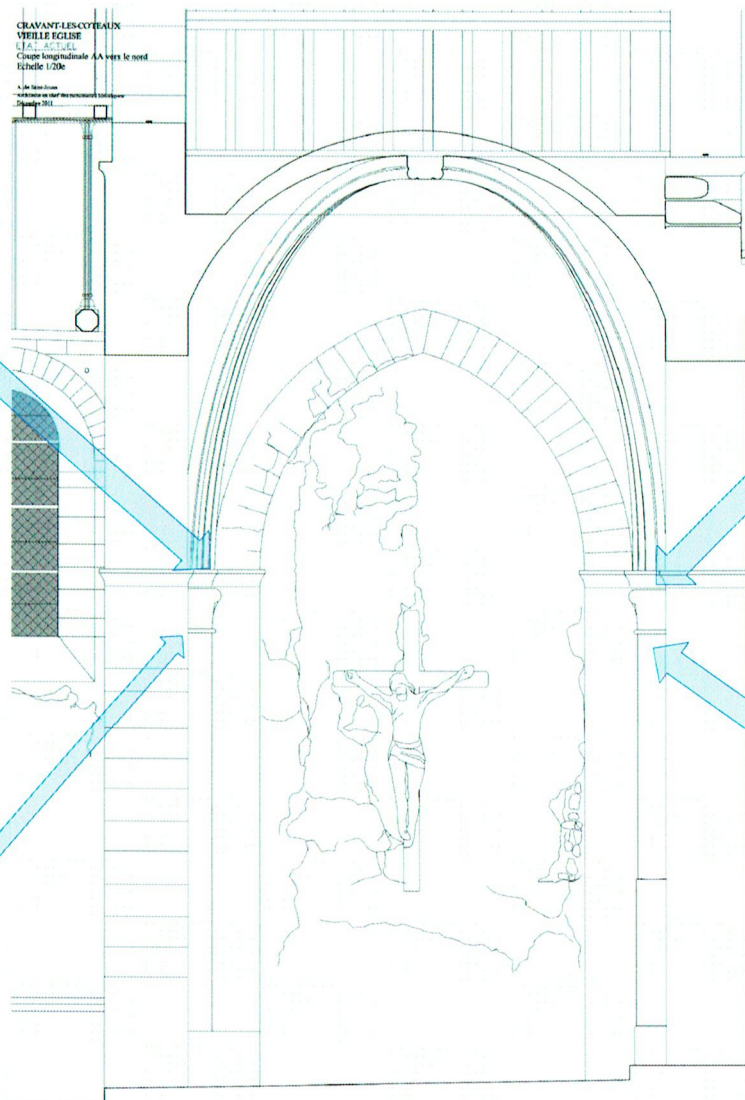
Elévation du mur Nord du transept (Plan de A. de Saint-Jouan)
